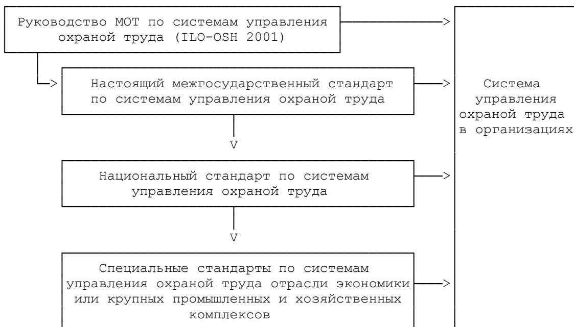
Рисунок 1. Элементы национальных структур систем управления охраной труда
