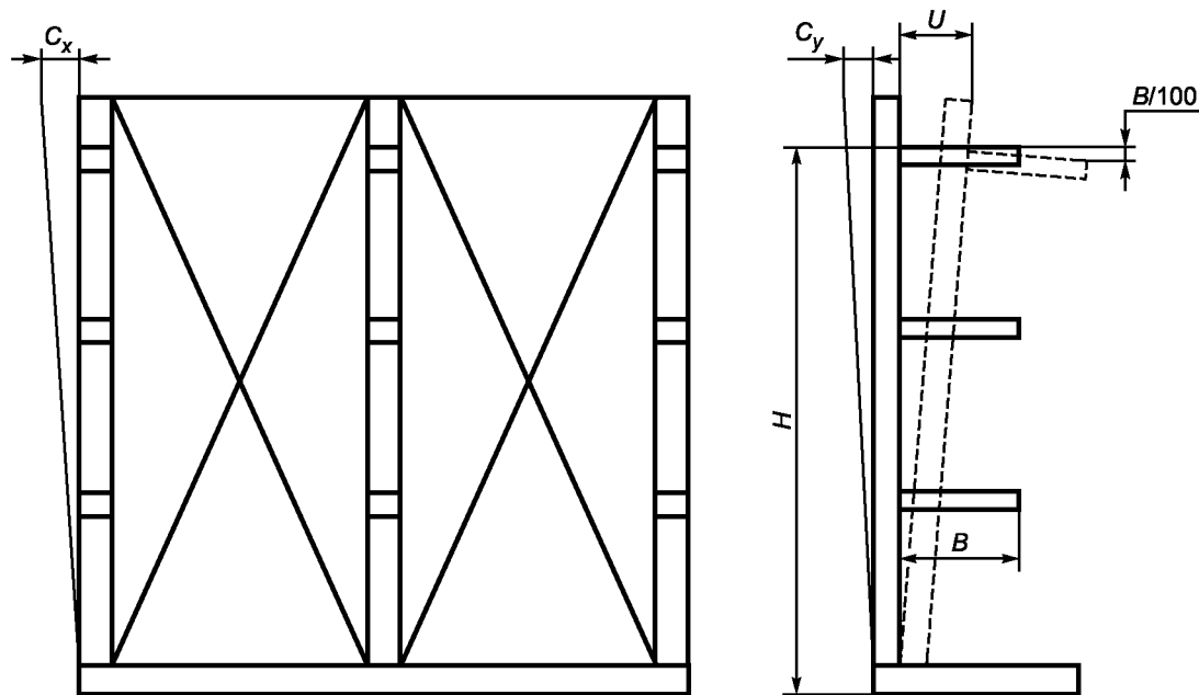
H — высота верхней консоли, B — длина консоли
