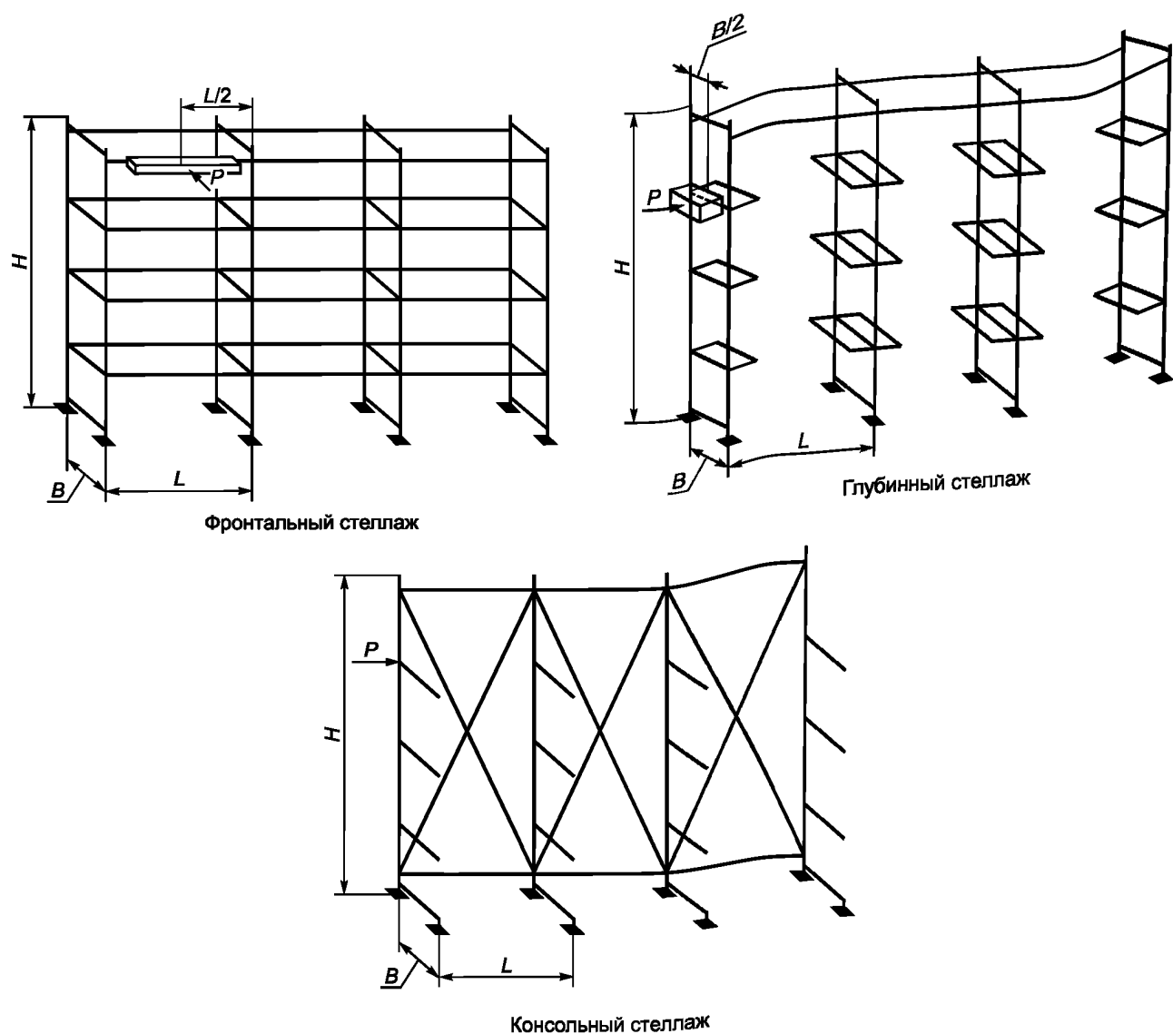
Рисунок 16 — Методы испытаний на воздействие горизонтальной нагрузки
